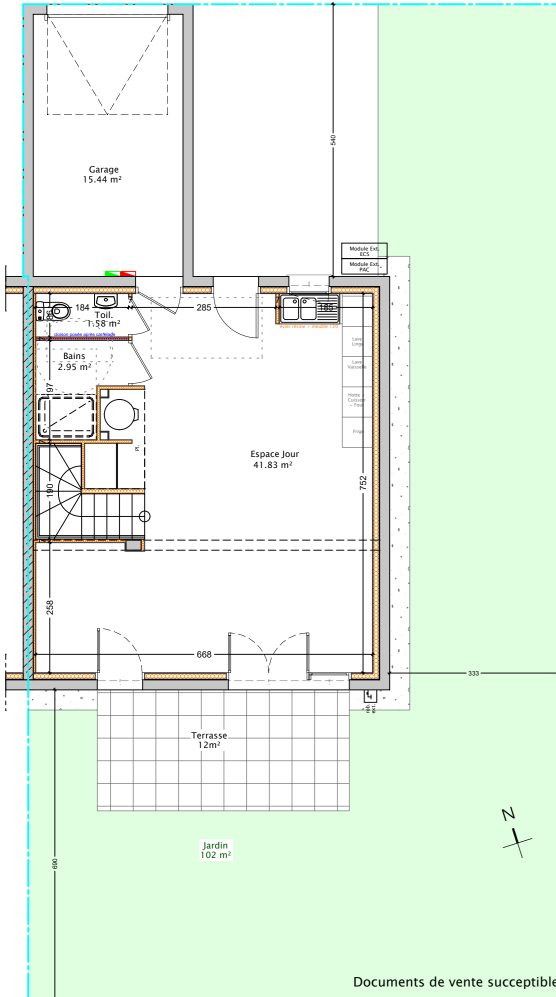
Plan Rez de Jardin – Ech. 1/75°
